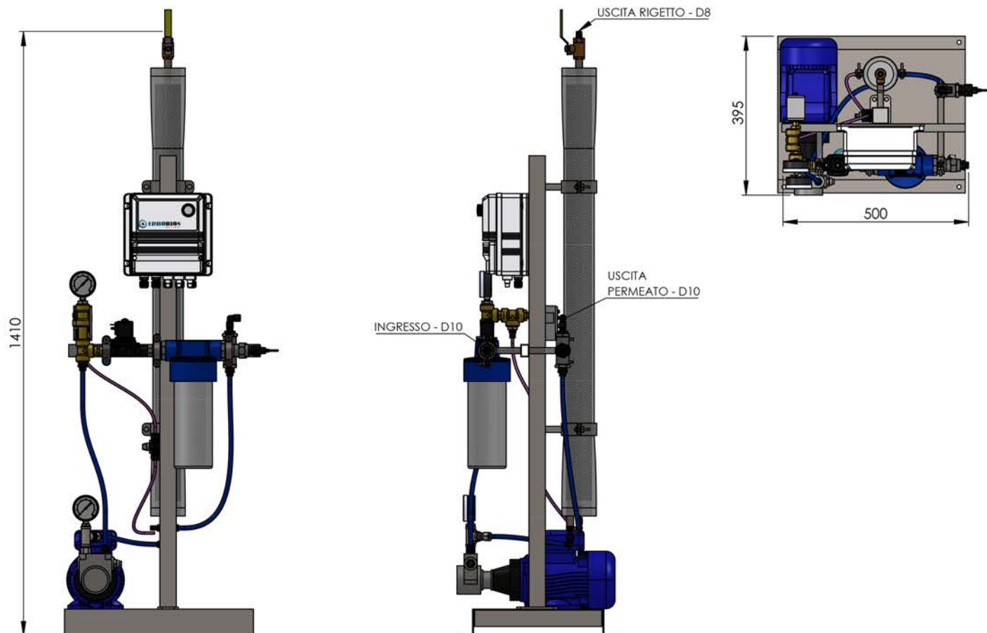
VISTA FRONTALE
